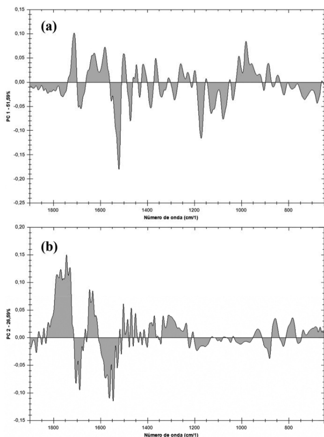
Figura 5. Loadings da componente principal 1 (a) e da componente principal 2 (b) para as amostras de lenhos carbonizados artificialmente em mufla para as três espécies de Araucariaceae avaliadas
