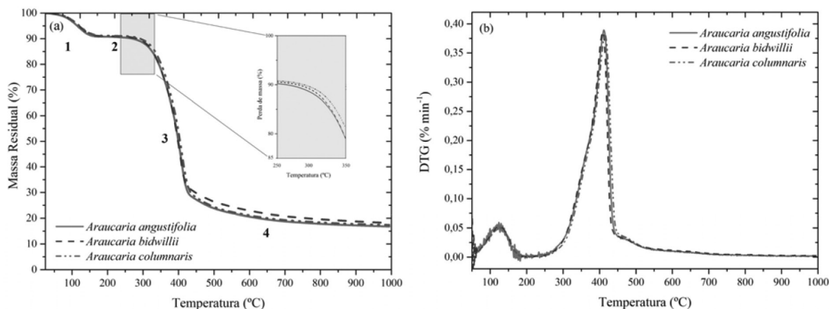
Figura 1. Medidas termogravimétricas das espécies Araucaria angustifolia , Araucaria bidwillii e Araucaria columnaris com razão de aquecimento de 25\text{ }^{\circ}\text{C min}^{-1} e faixa de temperatura de aquecimento de 25\text{ }^{\circ}\text{C} a 995\text{ }^{\circ}\text{C} (curvas TG) com regiões 1,2 (detalhe em zoom), 3 e 4 destacados (a) e curvas DTG (b)
