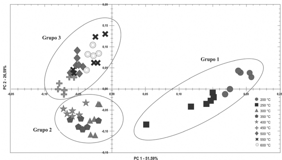
Figura 4. Representação dos scores para PC1 versus PC2 para as amostras de lenhos carbonizados artificialmente em mufla para a A. angustifolia , A. bidwillii e A. columnaris
