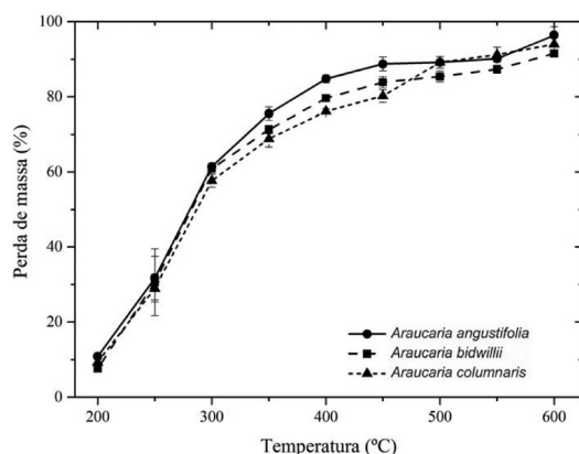
Figura 2. Perda de massa das amostras submetidas ao processo de queima em mufla para as espécies Araucaria angustifolia , Araucaria bidwillii e Araucaria columnaris na faixa de temperatura de 200 °C a 600 °C
