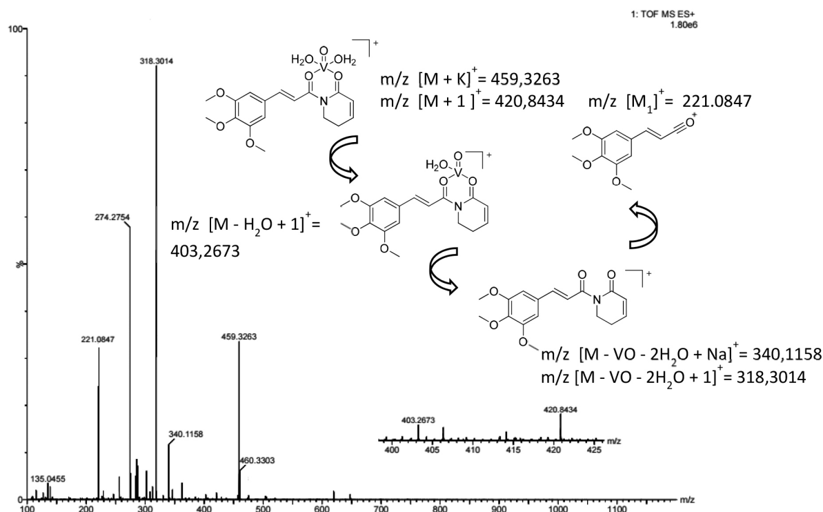
Figura 5. Espectro de massas do complexo V-PIP, analisado em modo positivo, com destaque no pseudo íon molecular [\text{VO}(\text{PIP})(\text{H}_2\text{O})_2 + \text{K}]^+
