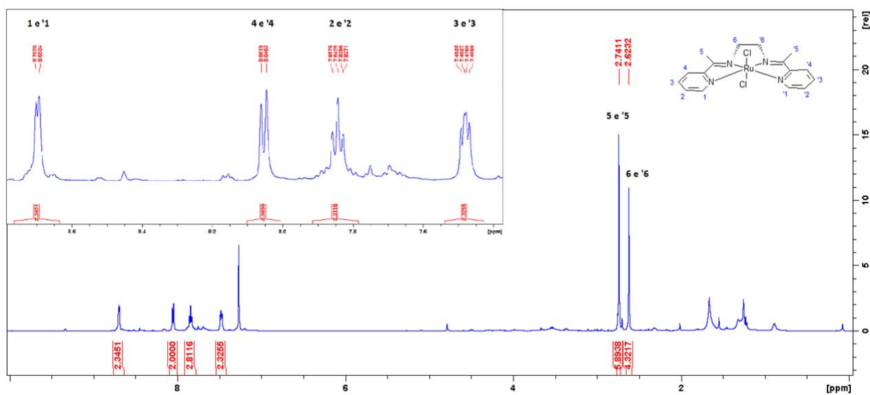
Figura 1S. Espectro de RMN de ^1\text{H} do complexo de rutênio dissolvido em clorofórmio deuterado
