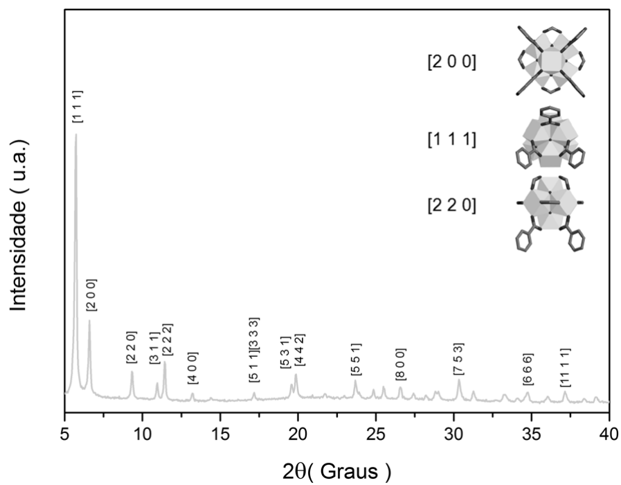
Figura 2S. Difratoograma de raios X, método do pó, da unidade metalo-orgânica MOF UiO-67, contendo os índices de Miller para planos da estrutura cúbica da MOF.
