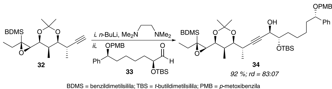
Esquema 18 - Controle Felkin-Anh na rota de síntese do sorafená A
