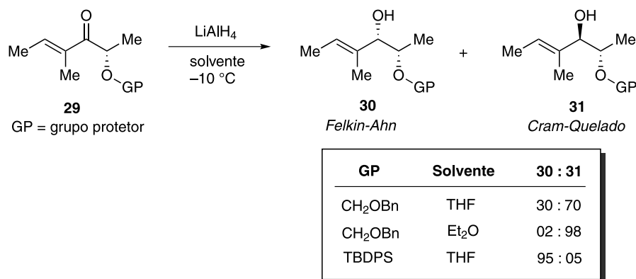
Esquema 17 - Seletividade na redução de cetonas: Felkin-Anh x Cram-quelado
