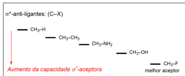
Figura 9 - Capacidade aceptor de ligações C-X
