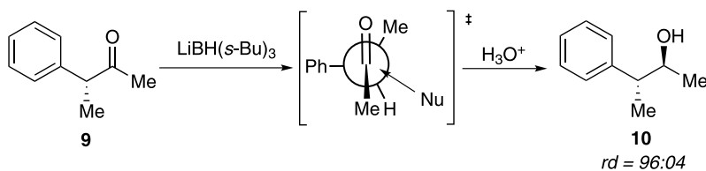
Esquema 9 - Redução diastereosseletiva da cetona 9
