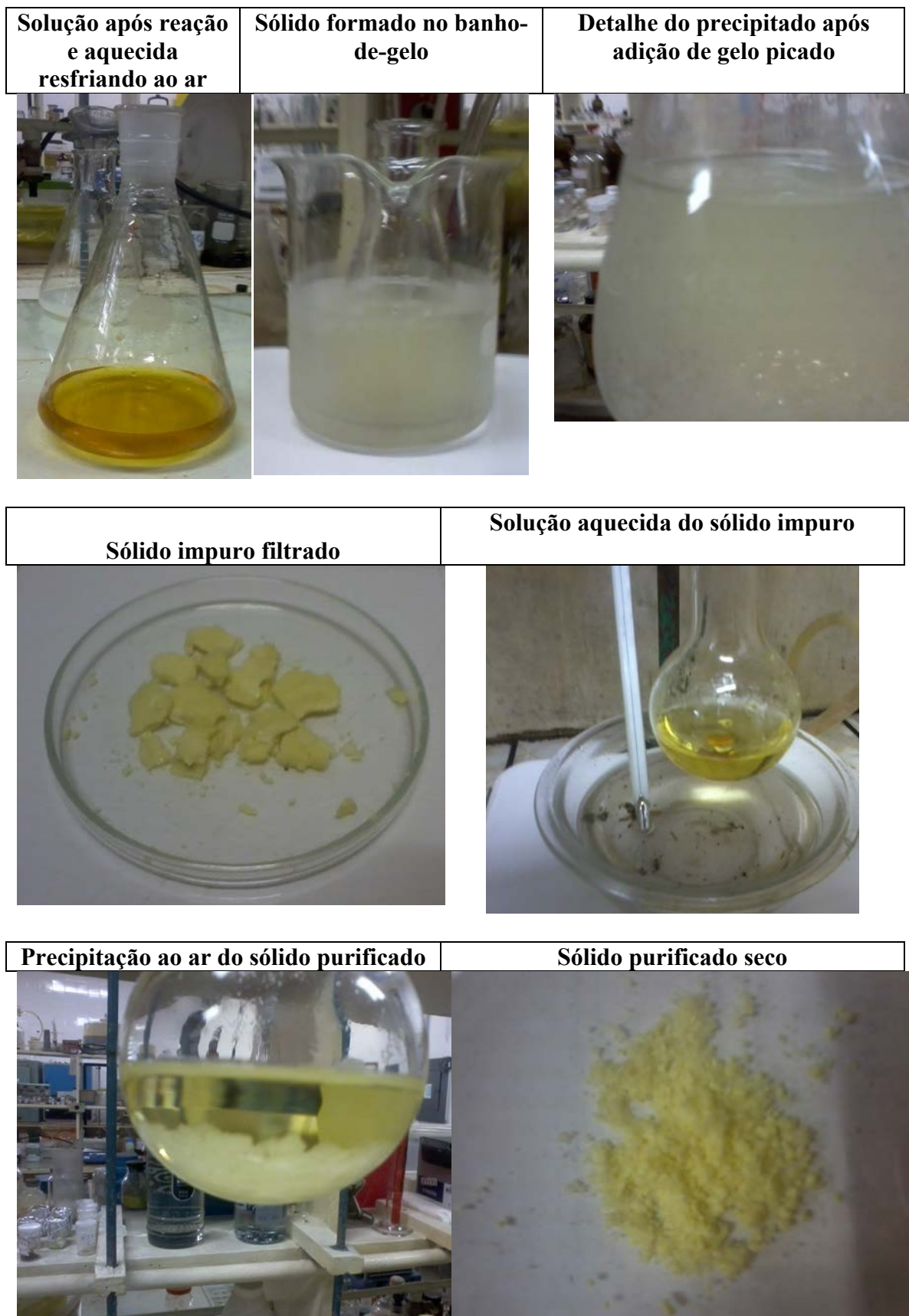
Figura 3S. Fotos da sequência da purificação da benzalacetofenona em cachaça
