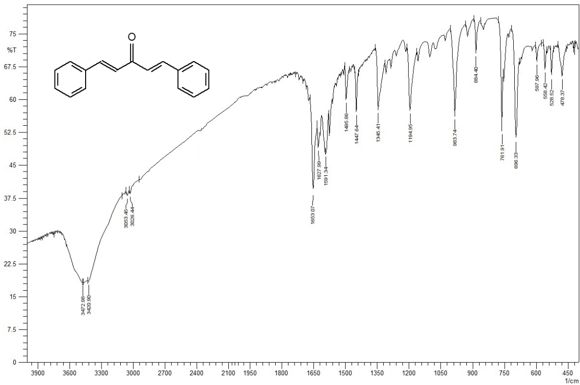
Figura 2S. Espectro na região do infravermelho (KBr) da dibenzalacetona obtida em cachaça
