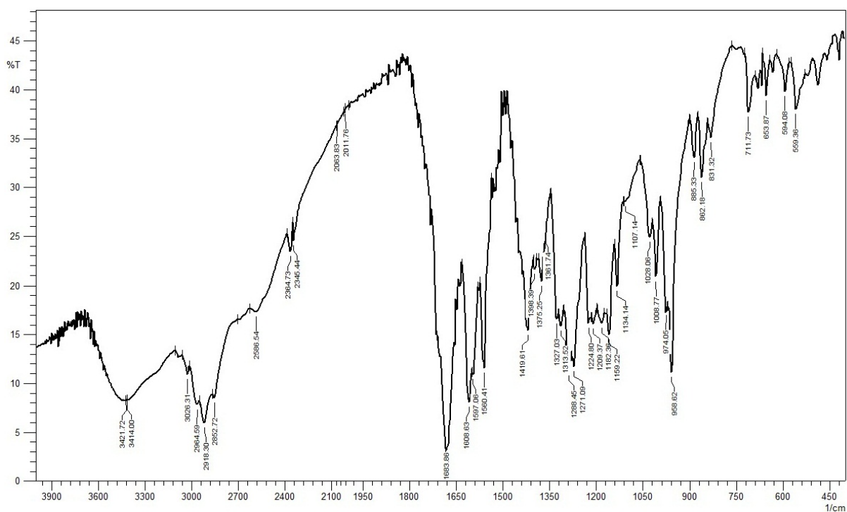
Figura 5S. Espectro na região do infravermelho (KBr) do pigmento de urucum obtido na extração com NaOH 5% em cachaça
