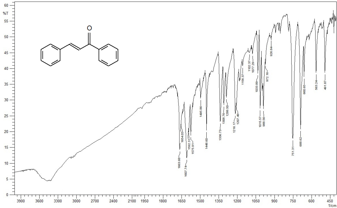
Figura 1S. Espectro na região do infravermelho (KBr) da benzalacetofenona obtida em cachaça
