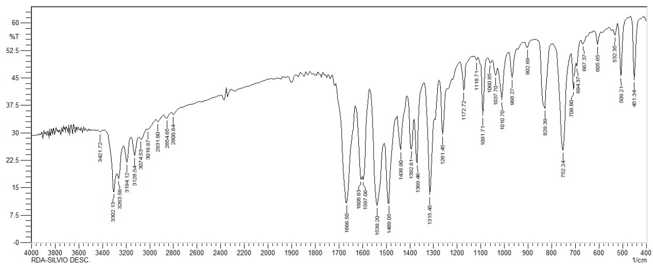
Figura 1S. Espectro na região do infravermelho (KBr) da 4-cloroacetanilida após recrystalizar
