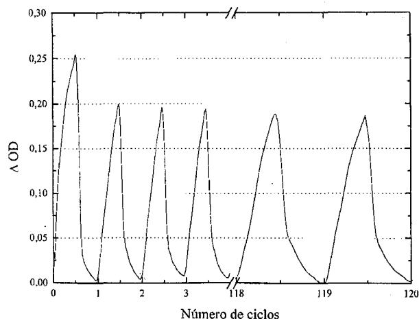
Figura 4. Mudança do \Delta OD de filme de Nb_2O_5 imerso em solução 0,1M de LiClO_4/PC em função de número de ciclos.
