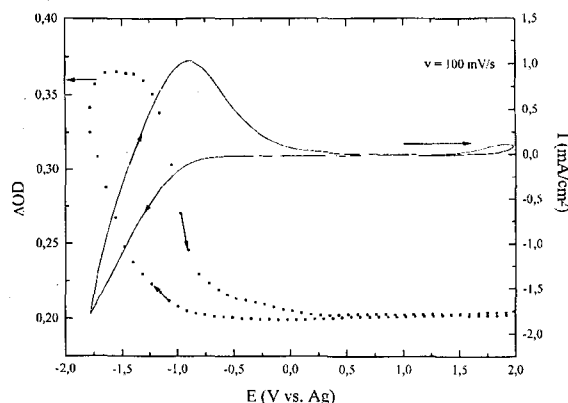
Figura 2. Voltametria cíclica (—) à 100mV/s de um filme de Nb 2 O 5 (espessura de ~300nm) tratado a 560 °C e ΔOD versus E (.....) para λ=600nm.
