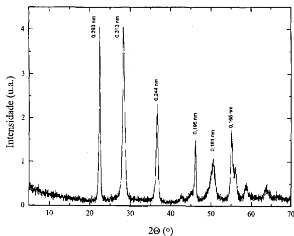
Figura 1. Difratograma de raios-X do xerogel de Nb 2 O 5 tratado a 560 °C.
