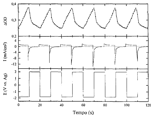
Figura 3. Gráfico de ΔOD e I(mA/cm 2 ) em função do tempo para ciclos cronoamperométricos de 10s e potenciais de -1,8V e 2,0V do filme de Nb 2 O 5 imerso numa solução de 0,1M de LiClO 4 /PC.
