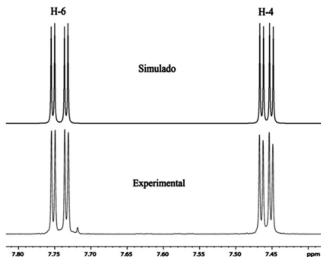
Figura 4. Comparação entre sinais de RMN de ^1\text{H} , simulado e experimental, para a substância 3
