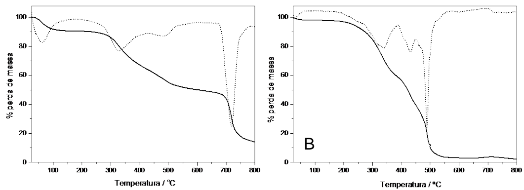
Figura 1S. Curvas TG (—) e DTG (---): (A)-PEDOT e (B)-MEH-PPV sob atmosfera de ar sintético
