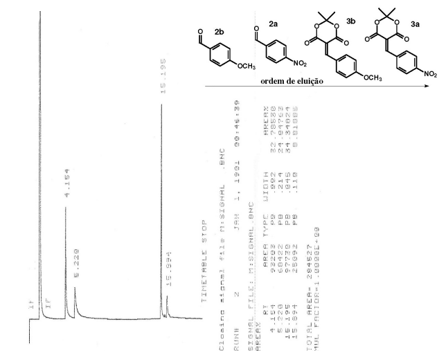
Figura 7S. Cromatograma 33 da mistura de padrões
